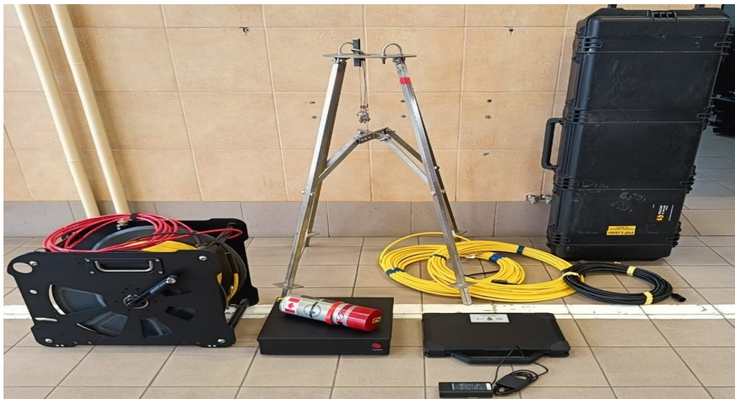
Sonar dookólny Imagenex 881A-GS
